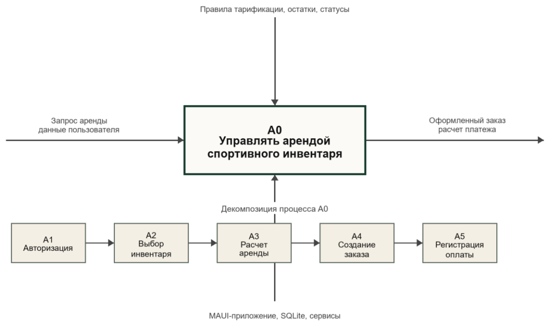
Рис. 4. Функциональная модель IDEF0 процесса аренды инвентаря
